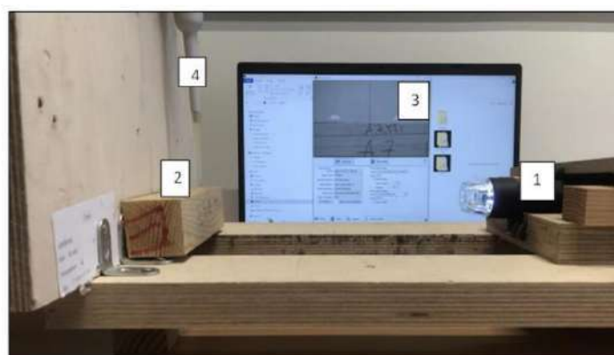
Figure 4 : Montage pour les mesures de tensions de surface. [1] Caméra, [2] Echantillon, [3] Ordinateur avec logiciel de commande de la caméra, [4] Pipette à coussins d'air
