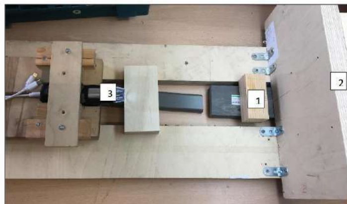
Figure 4 : Support pour les mesures d'impregnation et de tension de surface.
