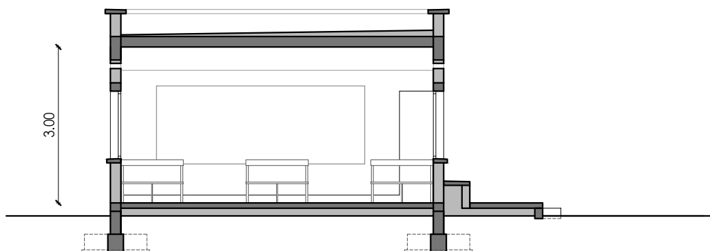
COUPE TRANSVERSALE
