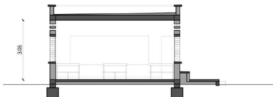
COUPE TRANSVERSALE
