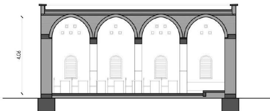
COUPE LONGITUDINALE 0 0.5 1 2 m
