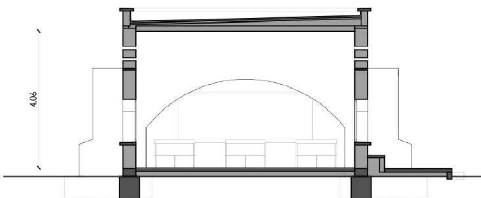
COUPE TRANSVERSALE 0 0.5 1 2 m
