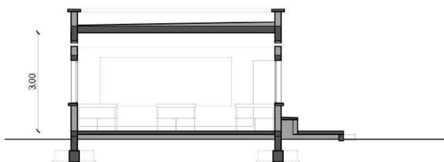
COUPE TRANSVERSALE
