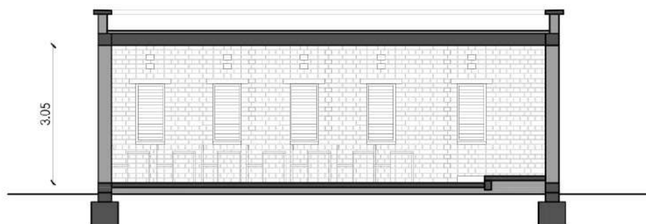
COUPE LONGITUDINALE
