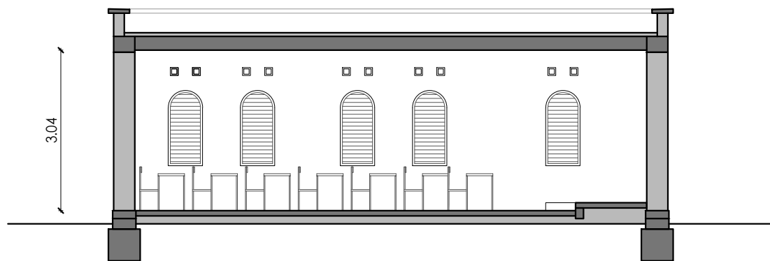
COUPE LONGITUDINALE
