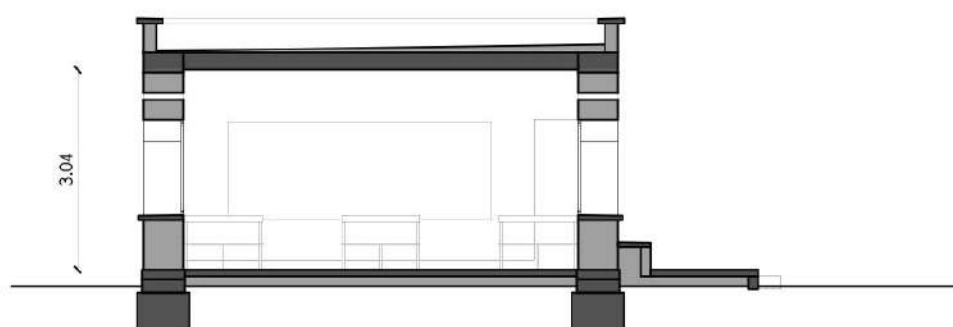
COUPE TRANSVERSALE 0 0.5 1 2 m
