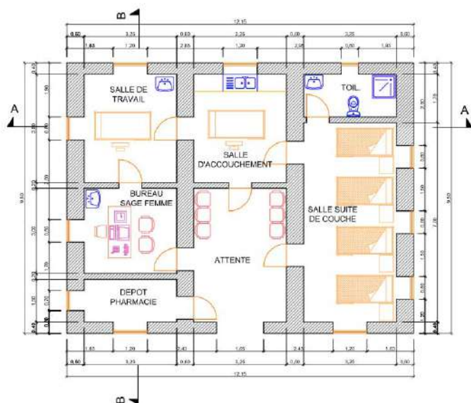
Plan architecturaux d'une maternité.
